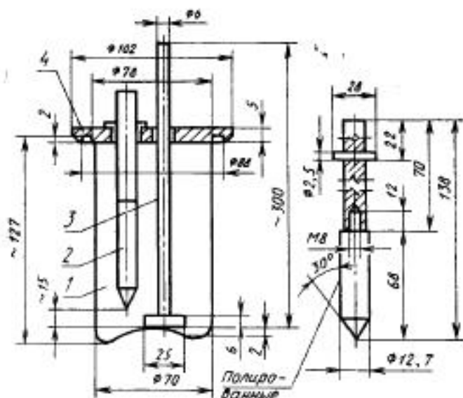
1 — стакан 2 — стержень; 3 — мешалка; 4 — крышка стакана
